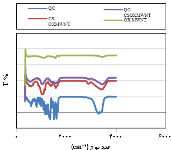
شکل ۱- طیف فروسرخ مربوط به نمونه‌های QC، CS-OXMWNT، QC-OXMWNT و QC-CSOXMWNT.
